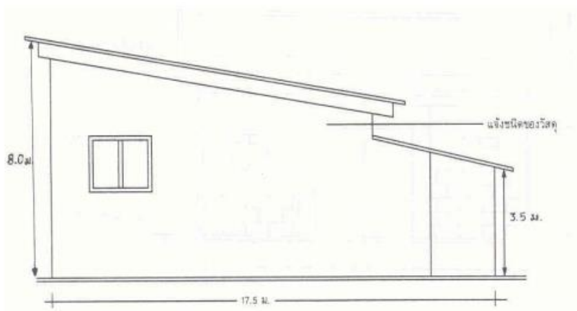
๓. ตัวอย่างแบบแปลนผนัง รูปด้านข้าง (ระบุมাত্রาส่วน วัสดุใช้สร้าง)
