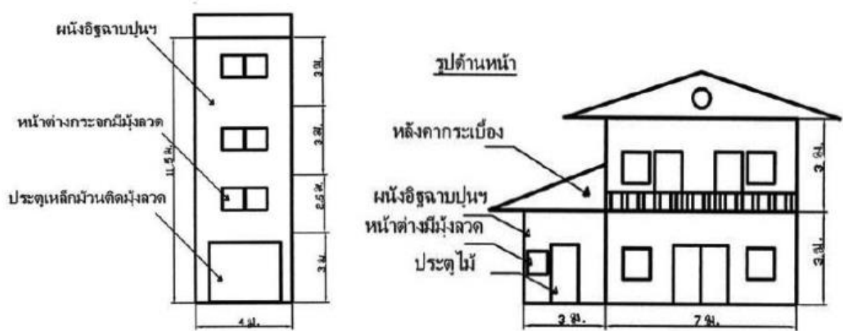
๓. ตัวอย่างแบบแปลนผนัง รูปด้านข้าง (ระบุมাত্রาส่วน วัสดุใช้สร้าง)
